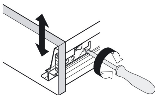
2. Justering lådfront i höjddled
